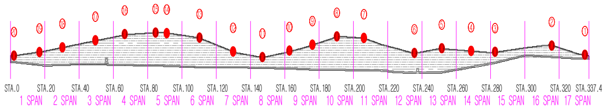
[수준측량 결과]
