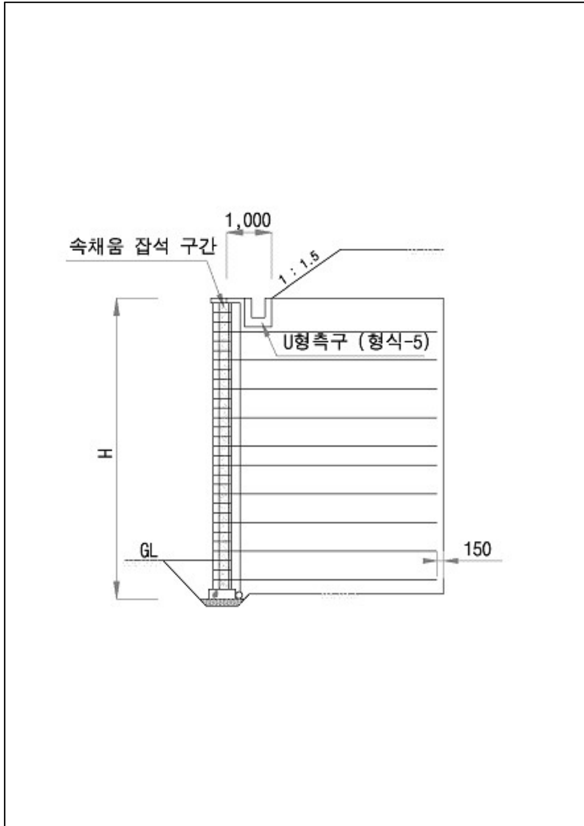
【그림 9.1.5】 표준 단면도
